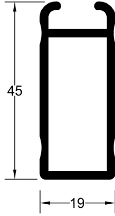
95-728 AĞIRLIK : 0.656 kg/mt.
