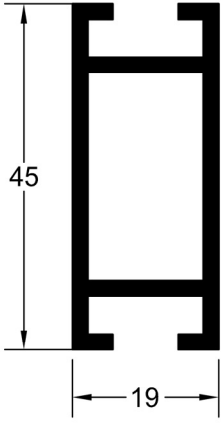
95-678 AĞIRLIK : 0.720 kg/mt.
