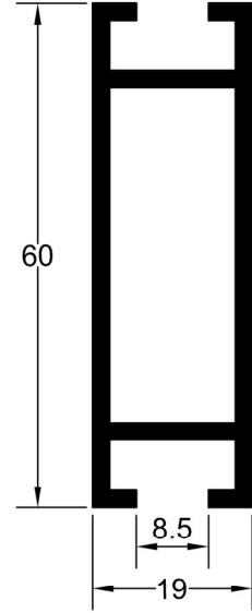
96-775 AĞIRLIK : 0.883 kg/mt.
