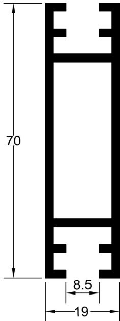
96-765 AĞIRLIK : 1.060 kg/mt.
