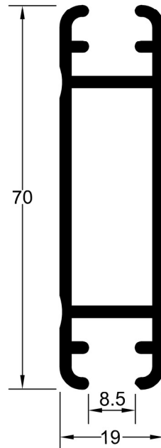
95-707 AĞIRLIK : 0.993 kg/mt.
