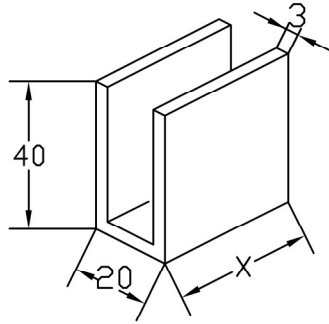
88-031 AĞIRLIK : 0.764 kg/mt.
