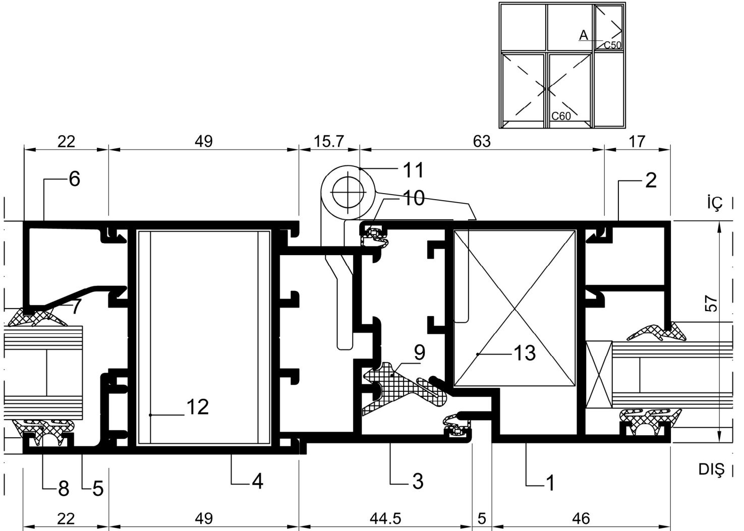
C60 sistemden C50 sisteme Geçiş Detayı
