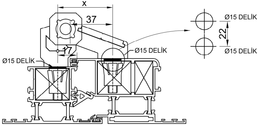
40 D 76 DIŞA AÇILIR MENTEŞE (YAYLI) (x = 54 mm)
