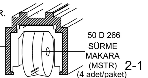
50 D 267 MAKARA TUTUCUSU (MSTR) (4 adet/paket)
