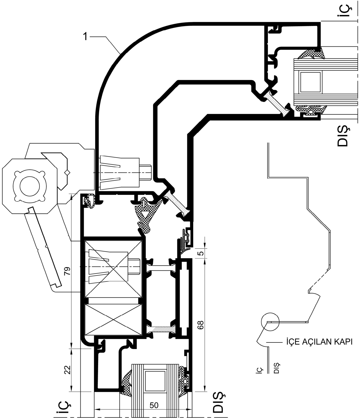
1. 90° İç Bükey Köşe Dönüş Profili 50 E 58
