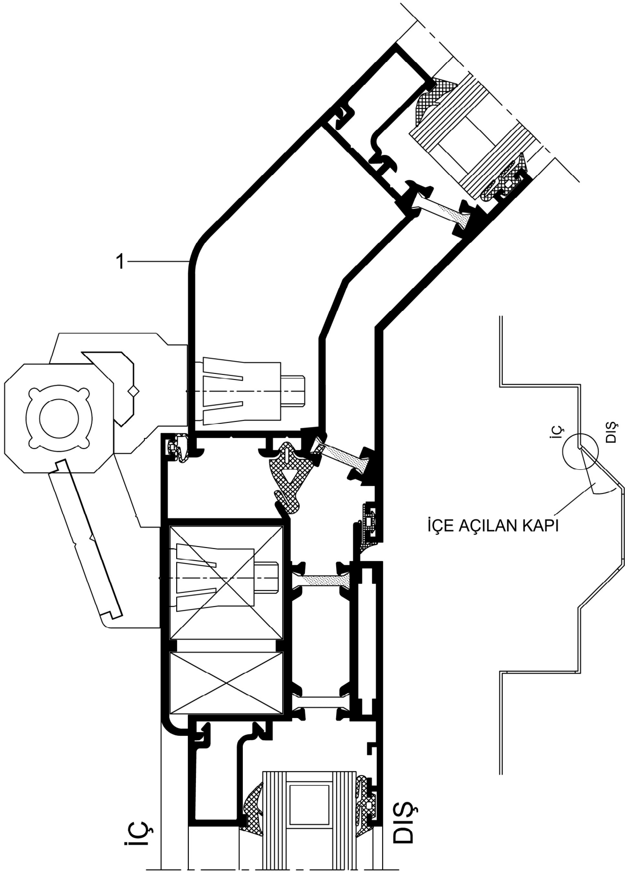
1. 135° İç Bükey Köşe Dönüş Profili
