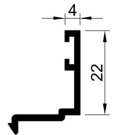
40 E 71 AĞIRLIK : 0.202 kg/m
