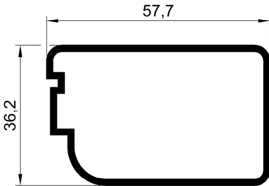
50 E 87 AĞIRLIK : 0.768 kg/m JX: 5.82 cm 4 JY: 12.15 cm 4
