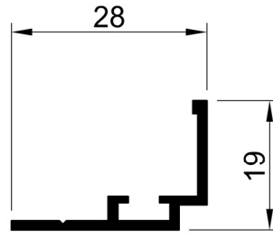
40 E 87 AĞIRLIK : 0.195 kg/m
