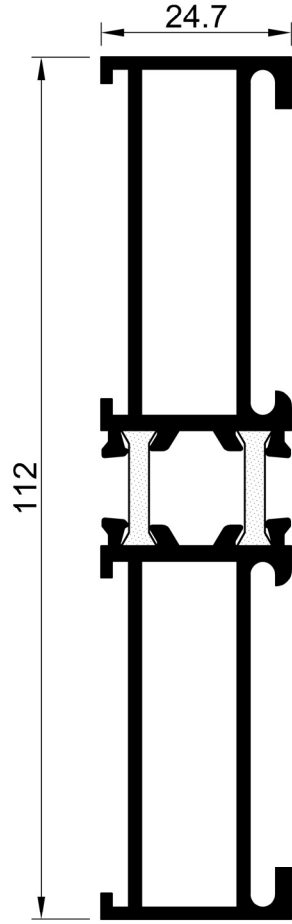
50 E 34 AĞIRLIK : 1.623 kg/m JX: 67.06 cm 4 JY: 3.33 cm 4
