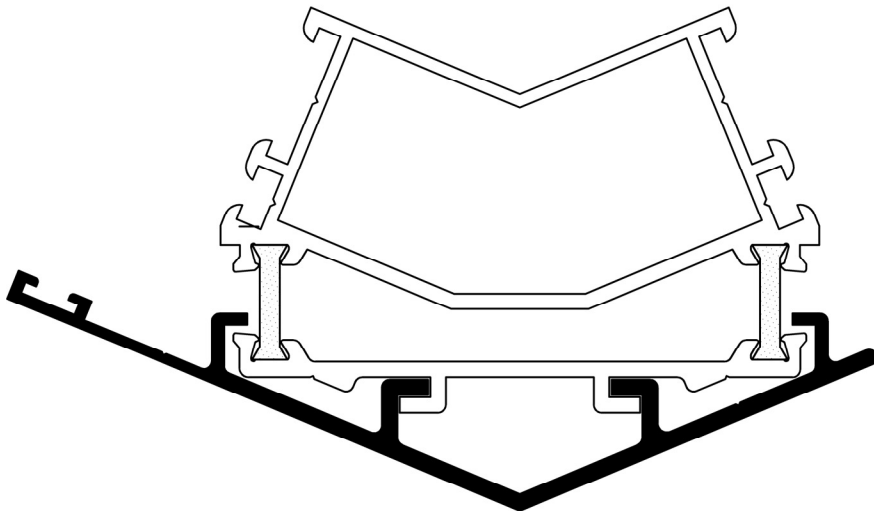
50 E 66 AĞIRLIK : 0.936 kg/m
