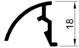
40 E 86 AĞIRLIK : 0.180 kg/m
