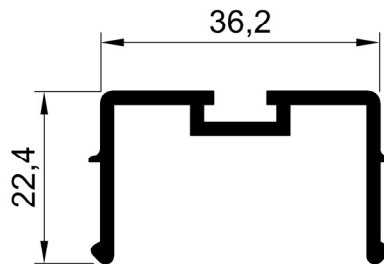
50 E 85 AĞIRLIK : 0.397 kg/m
