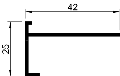
40 E 88 AĞIRLIK : 0.259 kg/m
