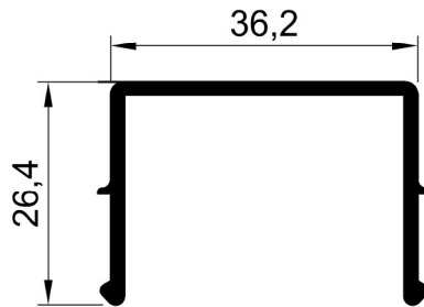
50 E 84 AĞIRLIK : 0.385 kg/m
