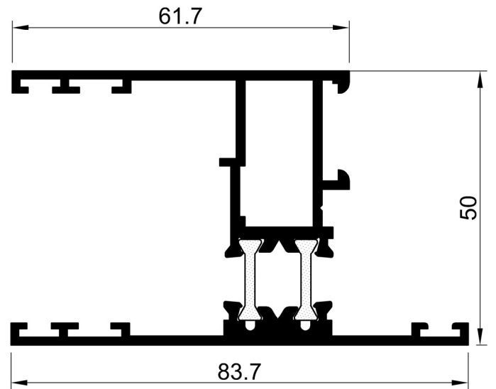
50 E 35 AĞIRLIK : 1.484 kg/m JX: 19.69 cm 4 JY: 18.47 cm 4
