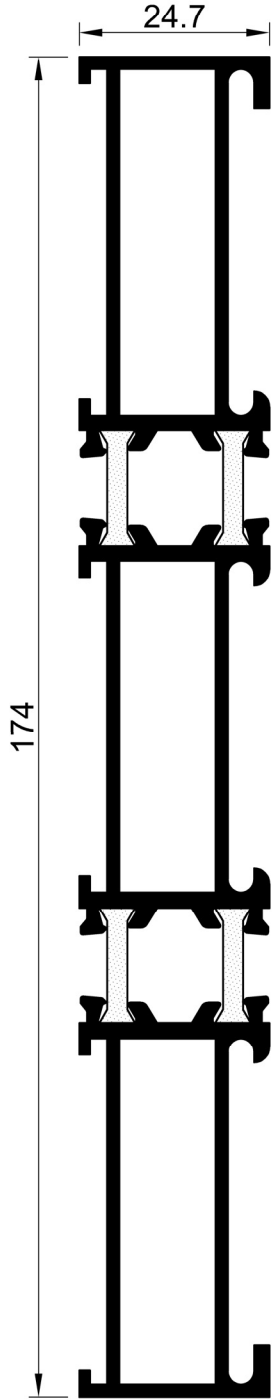
50 E 37 AĞIRLIK : 2.352 kg/m JX: 234.60 cm 4 JY: 5.18 cm 4
