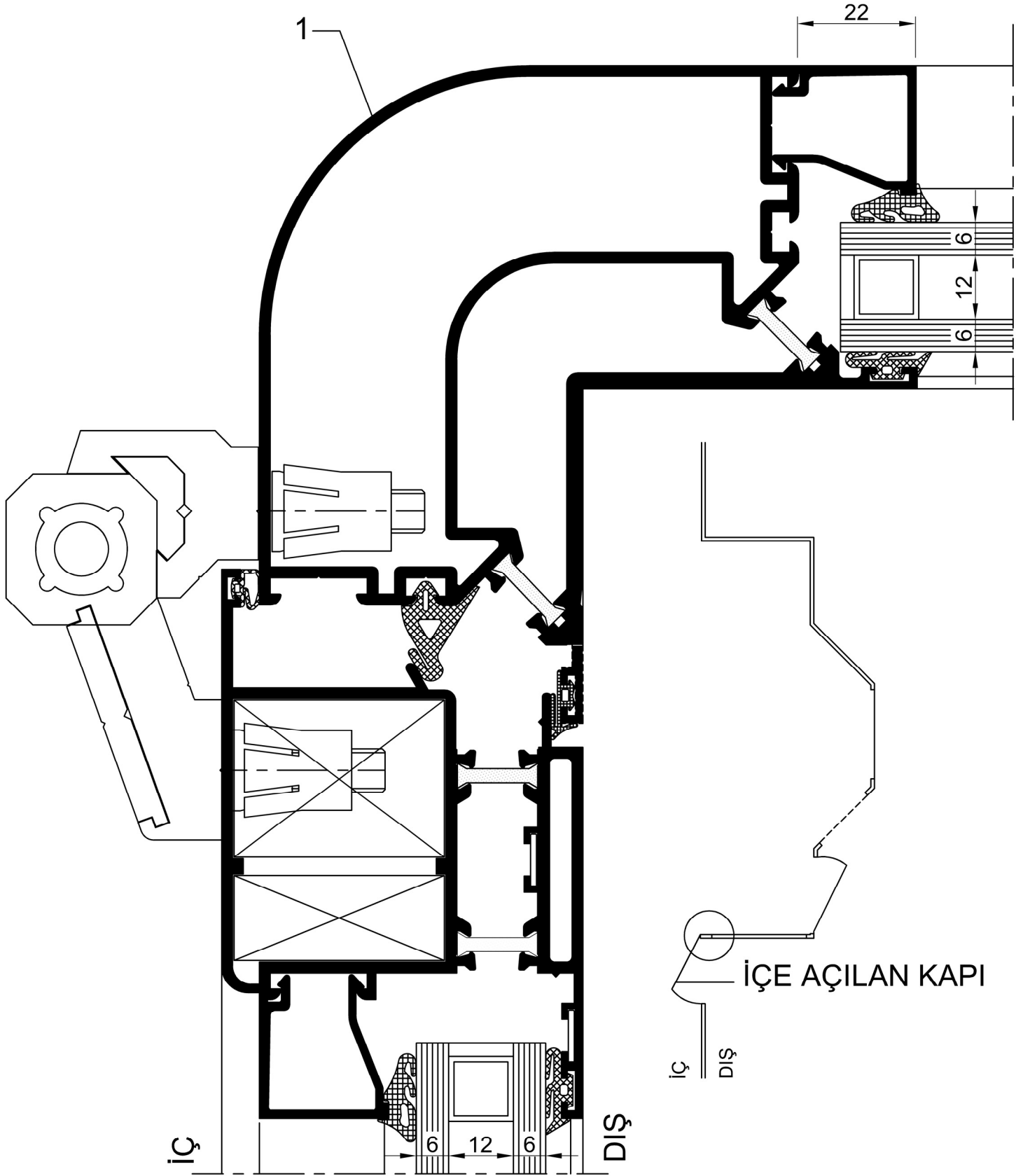
1. 90° İç Bükey Köşe Dönüş Profili 60 E 58
