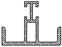
40 D 12 TOZ TUTUCU PLASTİĞİ (3 m)
