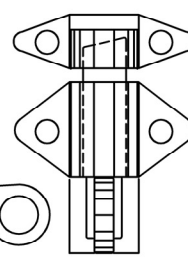
40 D 19 VASİSTAS ÇARPMA (HAM) (Eloksale Uygun Değildir) (adet) Ö:1/2
