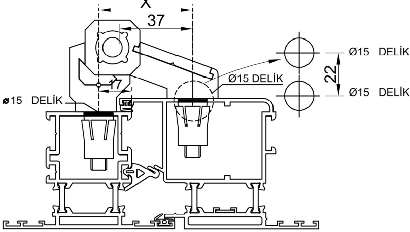
50 D 53 DIŞA AÇILIR MENTEŞE (YAYLI) (x = 54 mm) İÇE AÇILIR EGZANTRİK MENTEŞE (YAYLI) veya (DÜBELLİ) (x = 48 mm)
