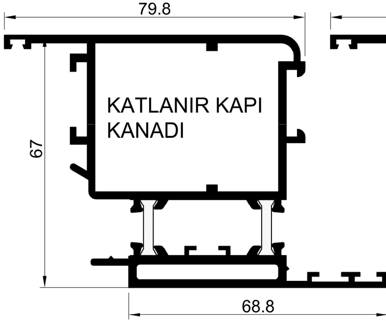
60 E 62 AĞIRLIK : 2.328 kg/m. JX: 49.02 cm 4 JY: 42.77 cm 4
