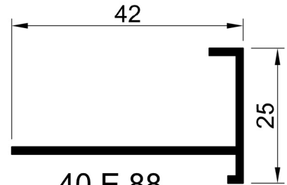
40 E 88 AĞIRLIK : 0.255 kg/m.
