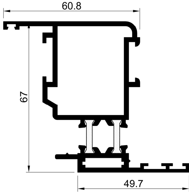
60 E 28 AĞIRLIK : 1.846 kg/m. JX: 38.13 cm 4 JY: 19.32 cm 4
