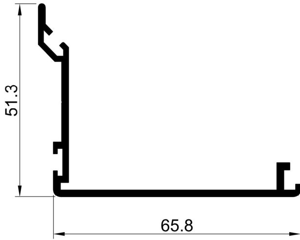
60 E 86 AĞIRLIK : 0.649 kg/m.
