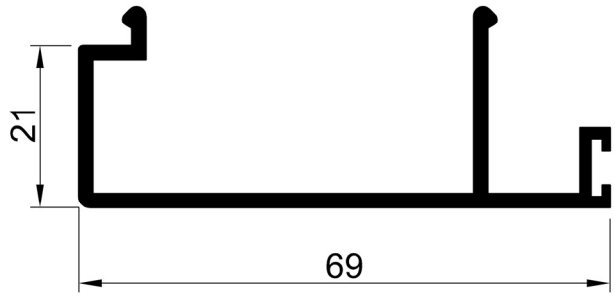
60 E 83 AĞIRLIK : 0.667 kg/m.
