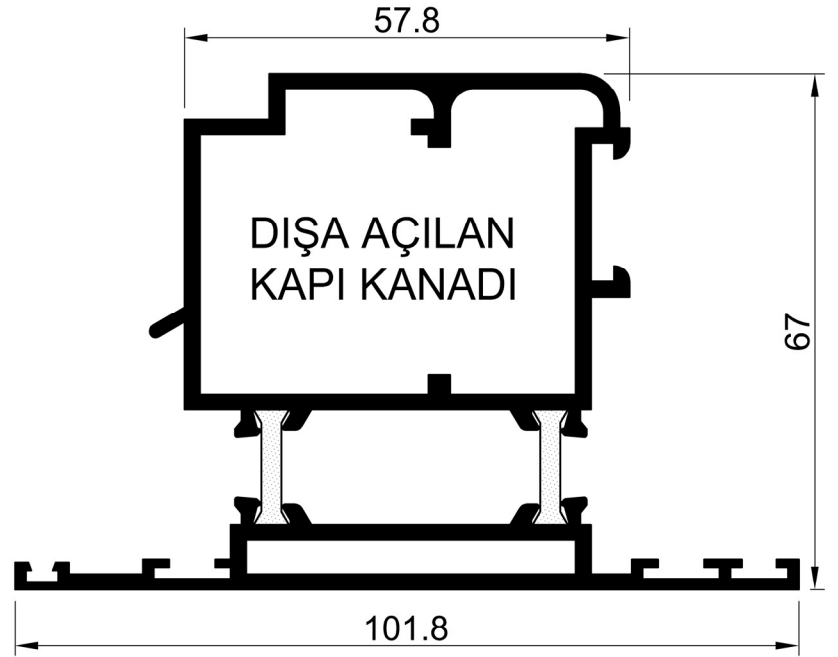
60 E 30 AĞIRLIK : 2.316 kg/m. JX: 47.10 cm 4 JY: 41.14 cm 4
