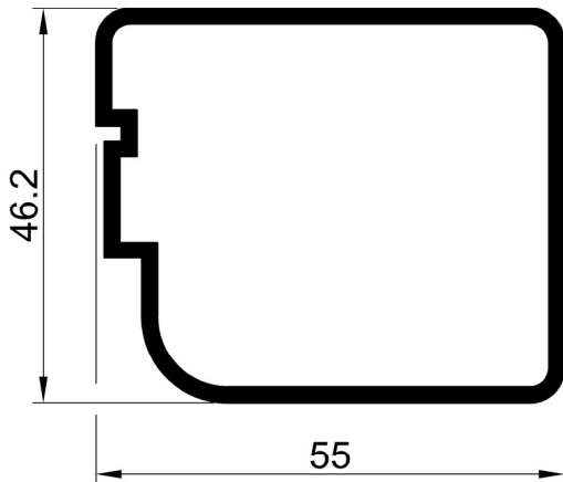
60 E 87 AĞIRLIK : 0.932 kg/m. JX: 10.86 cm 4 JY: 14.36 cm 4
