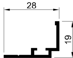
40 E 87 AĞIRLIK : 0.195 kg/m.
