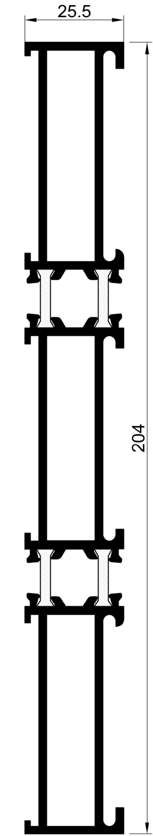
60 E 37 Ağırlık: 3.060 kg/m JX: 422.94 cm 4 JY: 6.78 cm 4
