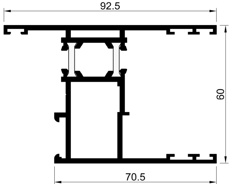
60 E 35 AĞIRLIK : 1.926 kg/m. JX: 36.36 cm 4 JY: 28.20 cm 4
