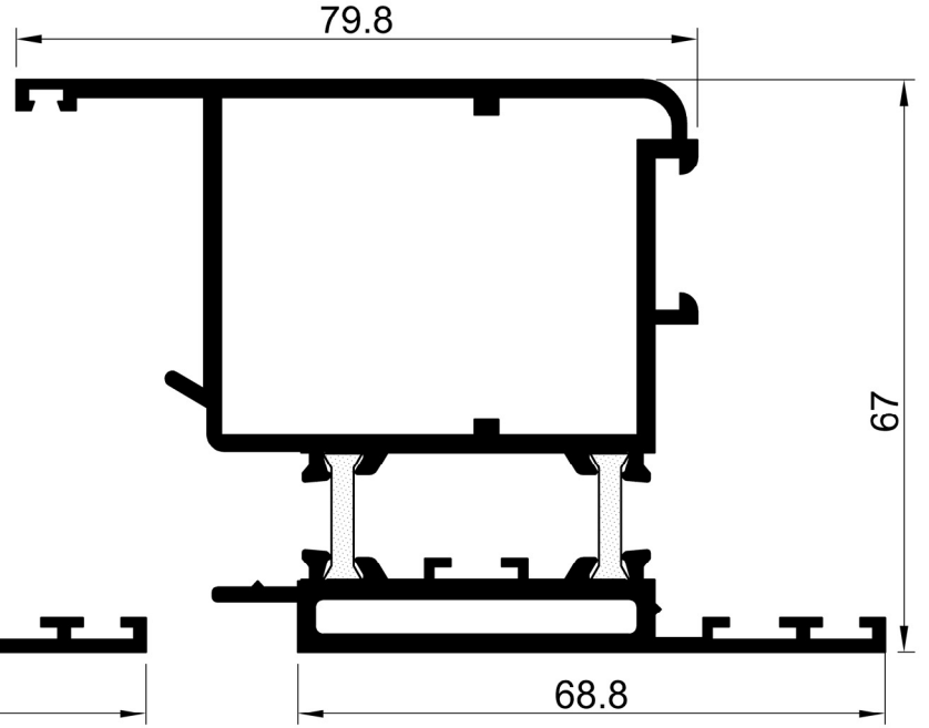
60 E 29 AĞIRLIK : 2.263 kg/m. JX: 47.77 cm 4 JY: 40.15 cm 4
