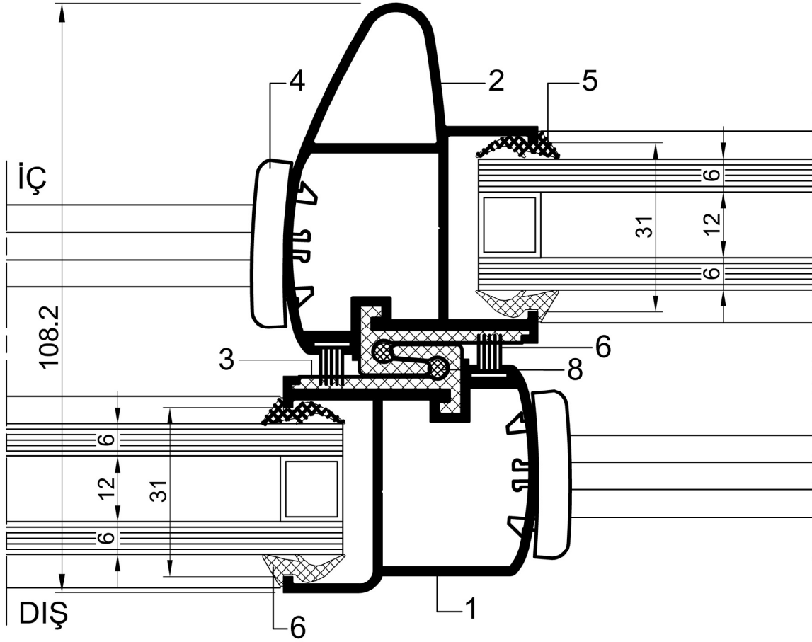
(2a) DETAYI
