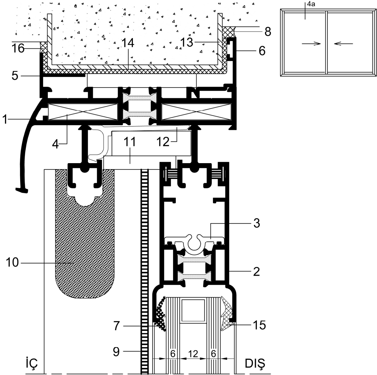
4a) DETAYI
