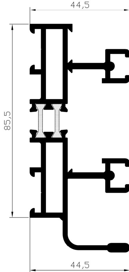
09-3034 Ağırlık: 2.300 kg/m
