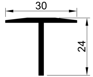
04-2166 Ağırlık: 0.260 kg/m
