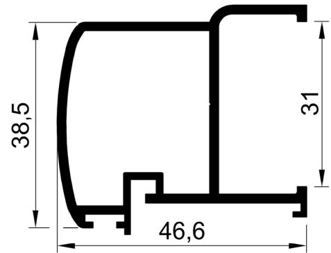
05-2329 Ağırlık: 0.756 kg/m
