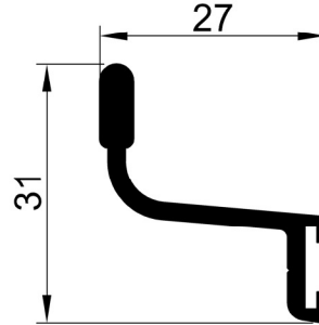
02-1839 Ağırlık: 0.355 kg/m
