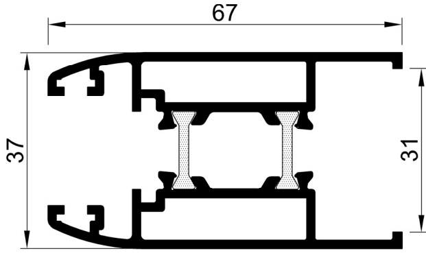
05-2331 Ağırlık: 1.340 kg/m
