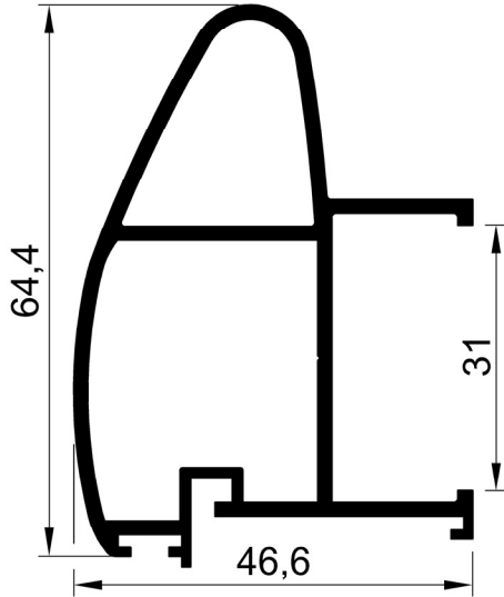
07-2595 Ağırlık: 1.014 kg/m
