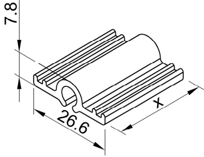
05-2332 Ağırlık: 0.231 kg/m
