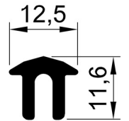
05-2333 Ağırlık: 0.168 kg/m
