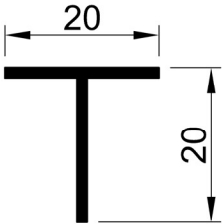
88-085 Ağırlık: 0.136 kg/m
