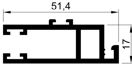
02-1732 Ağırlık: 0.674 kg/m
