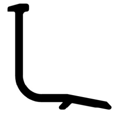
05-2335 Ağırlık: 0.251 kg/m
