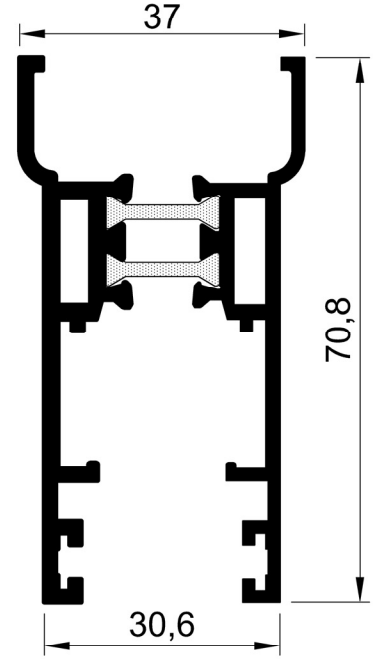
05-2334 Ağırlık: 1.282 kg/m
