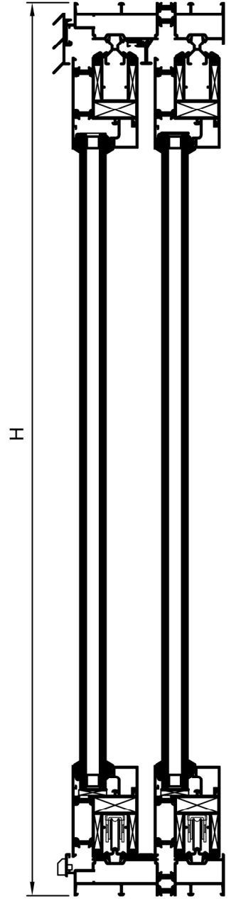
B-B Kesiti Section B-B
