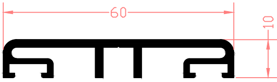
90-239 Ağırlık: 0,602 kg/mt
