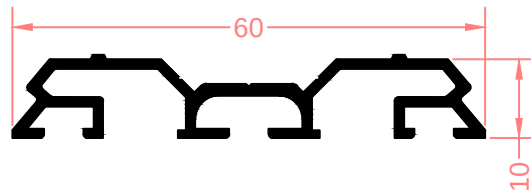
05-2345 Ağırlık: 0,443 kg/mt
