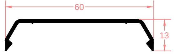
05-2344 Ağırlık: 0,282 kg/mt
