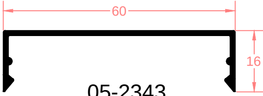
05-2343 Ağırlık: 0,334 kg/mt
