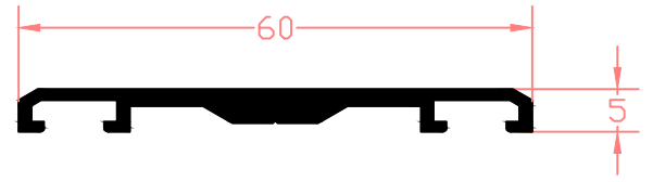
90-240 Ağırlık: 0,421 kg/mt
