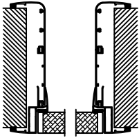
B-B Kesiti
