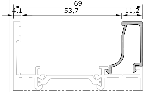
9047 11,2 mm Cam Çıtası 0,270 kg/m
