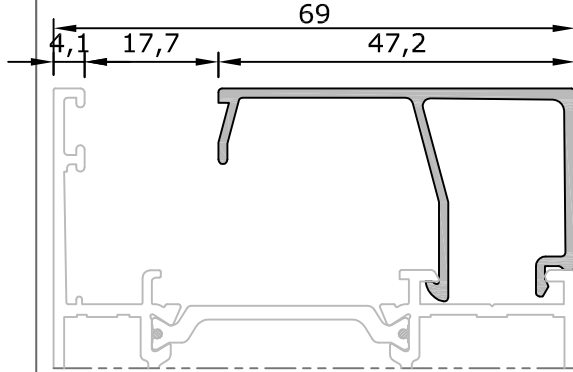
9073 47,2 mm Cam Çıtası 0,415 kg/m
