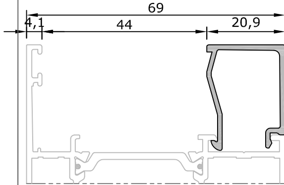
9074 20,9 mm Cam Çıtası 0,300 kg/m
