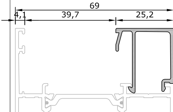
9044 25,2 mm Cam Çıtası 0,340 kg/m
