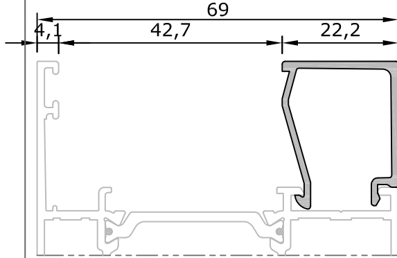
9048 22,2 mm Cam Çıtası 0,305 kg/m
