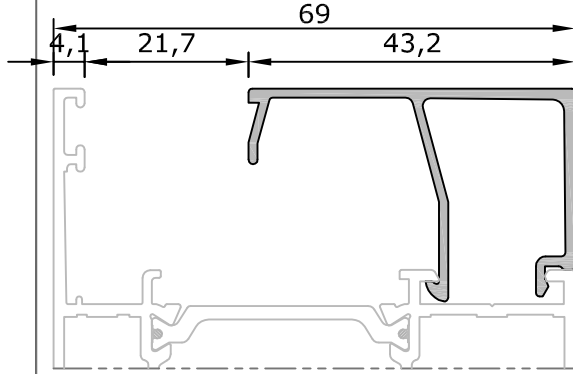
9072 43,2 mm Cam Çıtası 0,400 kg/m
