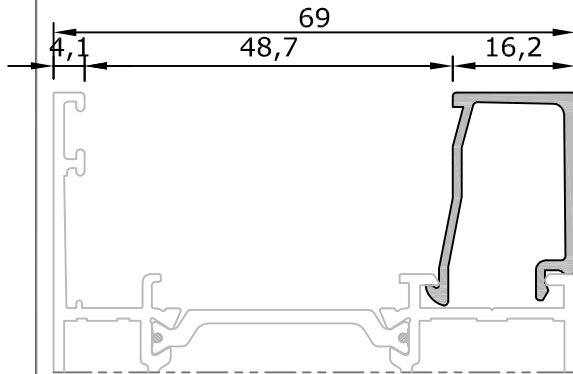
9045 16,2 mm Cam Çıtası 0,280 kg/m
