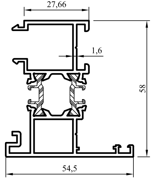
No:5556/57 Çift Kapı Adaptörü 1,285 kg/m
