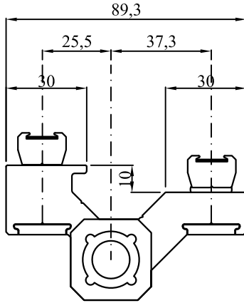
No : 312 - 313 - 314 Fugalı Kapazlama Mentеше ( 10 Adet / Paket )
