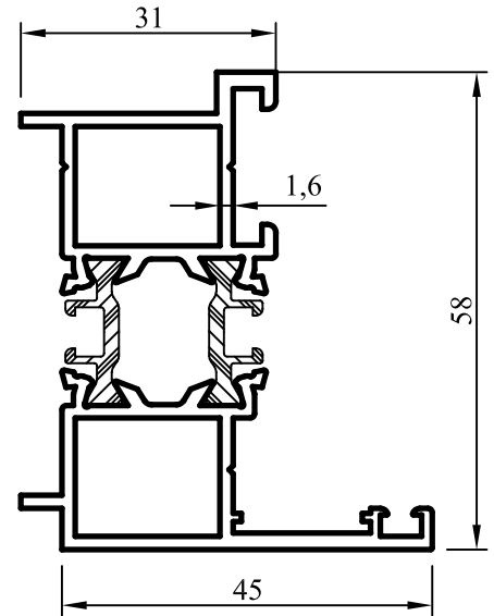
No:5558/59 Dışa Açılır Kapı Adaptörü 1.225 kg/m
