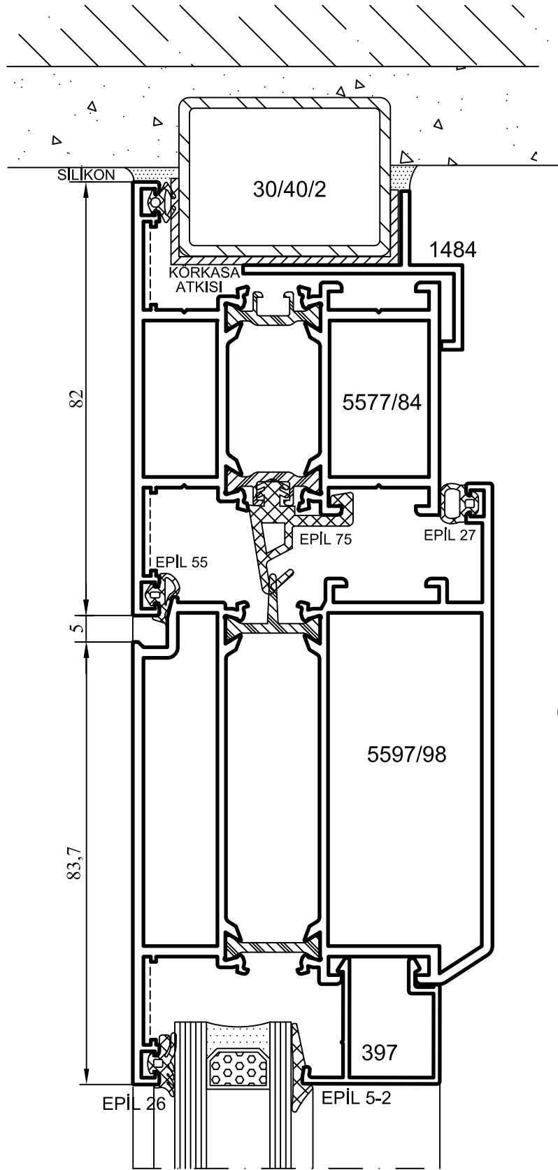
İÇE AÇILIR KAPI DOOR - INSIDE OPENING
