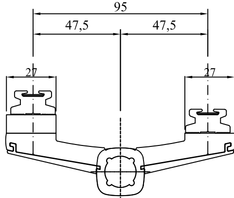
Kod : SFKM-58-077 Fugalı Kapazlama Mentеше ( 10 Adet / Paket )
