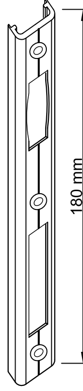
No : 7240-M Makaralı Kilit Karşılığı ( İstenilen Miktarda )
