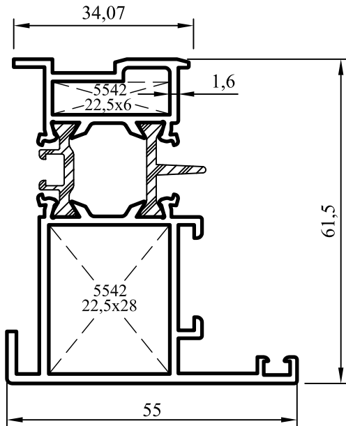
No:5562/63 Pivot Adaptörü 1,390 kg/m
