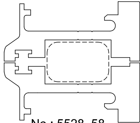
No : 5528_58 Pivot Mentеше 58 ( 2 Adet / Paket )
