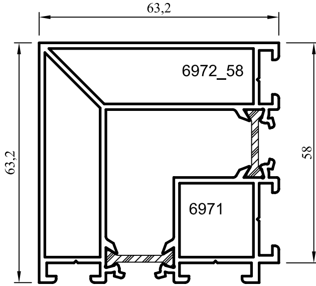
No:6971/72_58 90° Köşe Dönüş Profili 1,950 kg/m
